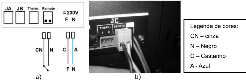
Figura 32 - Ligação do comando remoto sem fios
