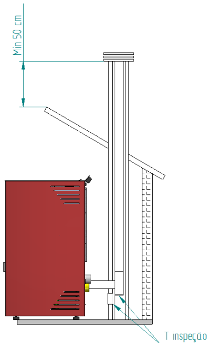
Figura 8 – Vista lateral da instalação com chaminé, com exemplo do ponto de inspeção
