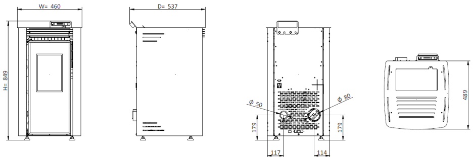
Figura 3 – Dimensões da salamandra a pellets PS008.
