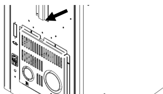
Figura 30 - Local onde é instalada a placa interface
