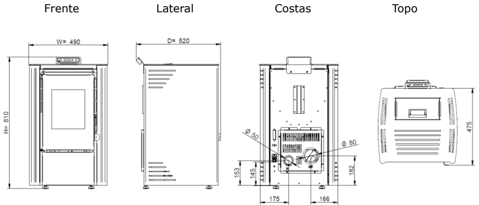
Figura 2 – Dimensões da salamandra a pellets First 6 kW.
