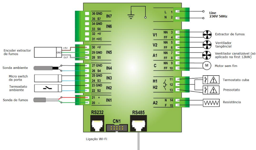
Figura 37 - Esquema elétrico (eletrônica Columbus)
