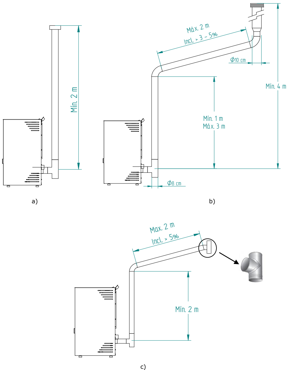
Figura 7 – Exemplos de instalações tipo
