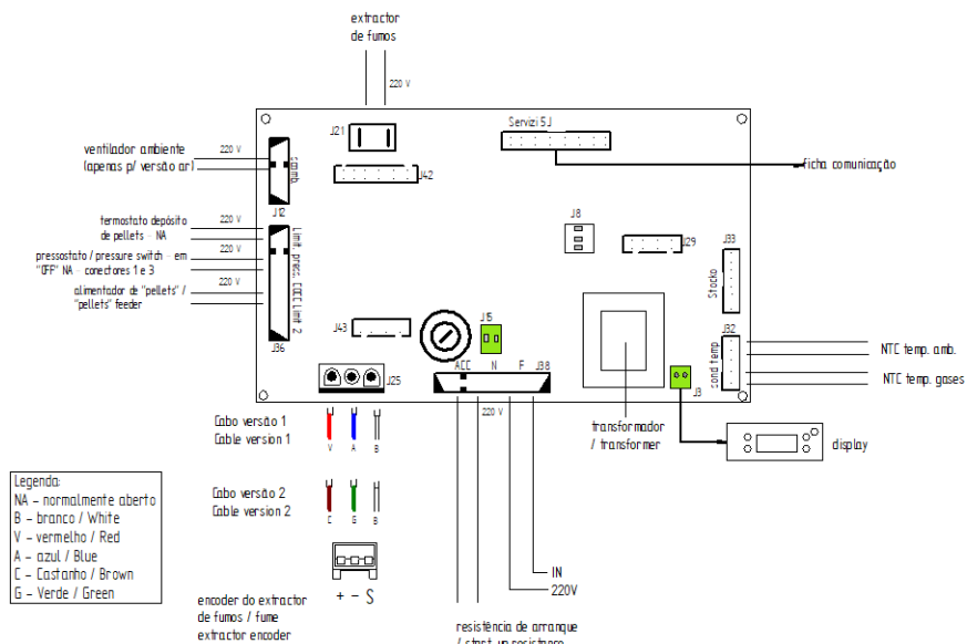
Figura 36 - Esquema elétrico
