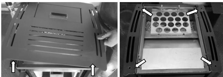
Figura 16 - Remoção tampo superior
